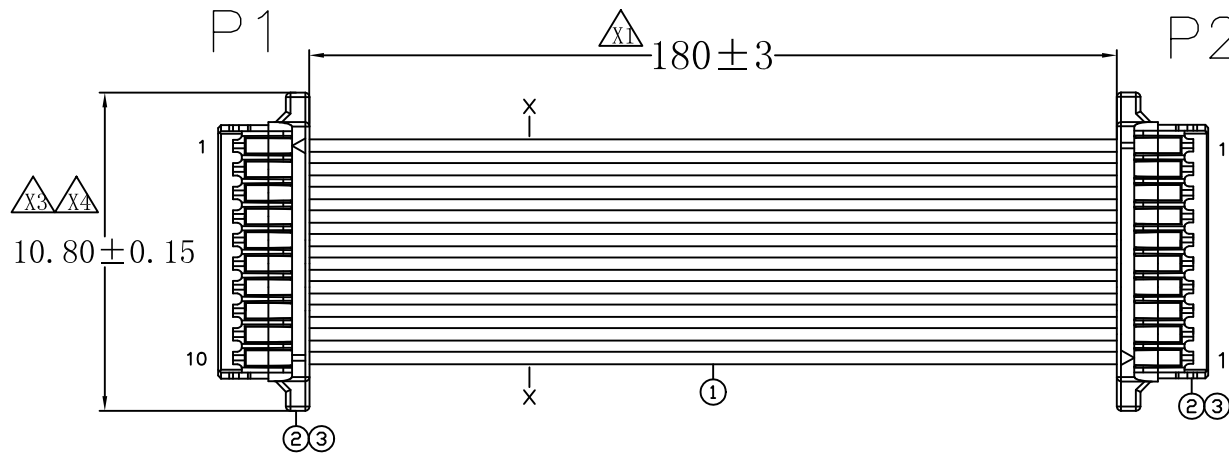
WIRING TABLE
